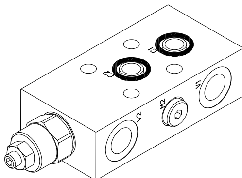
Versione corpo in acciaio Steel body version
